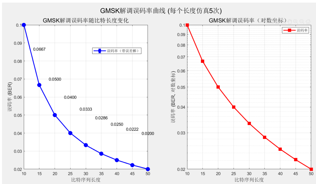
图 4-13 GMSK 误码率随比特数变化曲线
