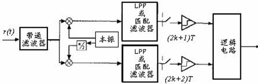
图 2-6 相干解调器
