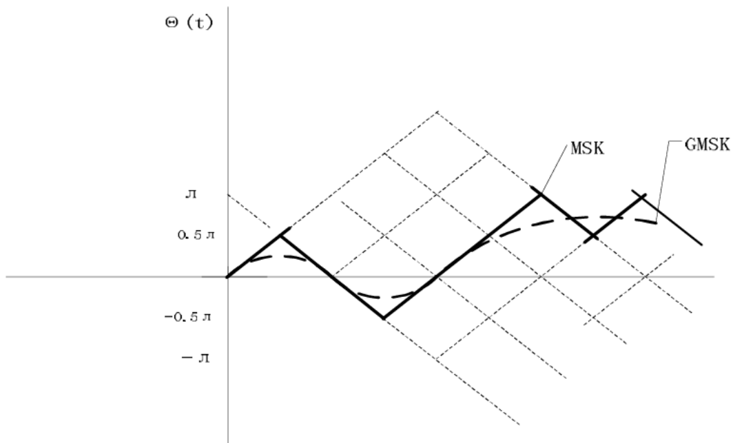
图 2-3 GMSK 相位路径图
